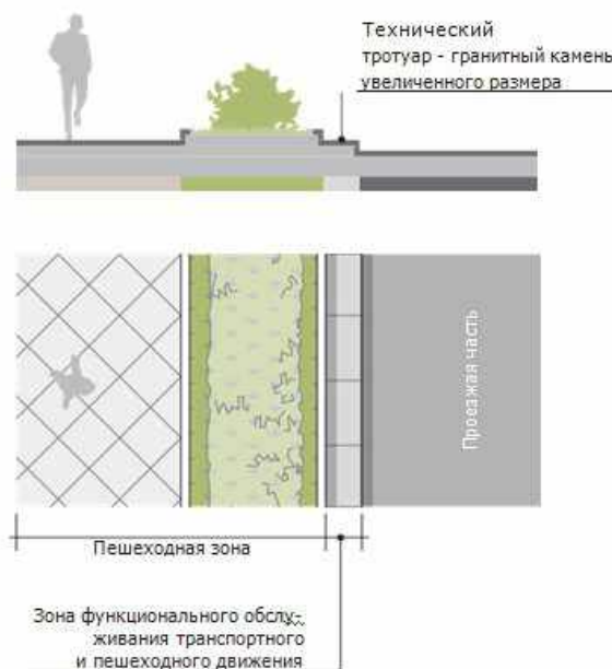
Технический тротуар, примыкающий к пешеходному тротуару на одном уровне
