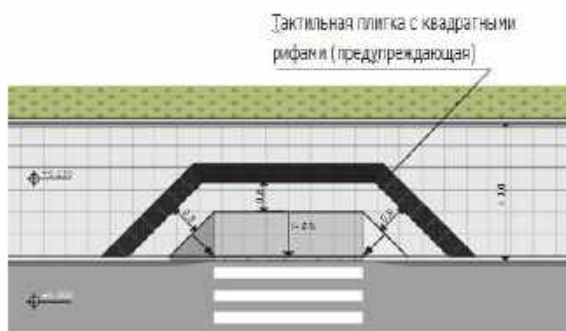
Схема 3. Наземный пешеходный переход. Ширина пешеходного тротуара — более 3,0 м. Размещение тактильных указателей
