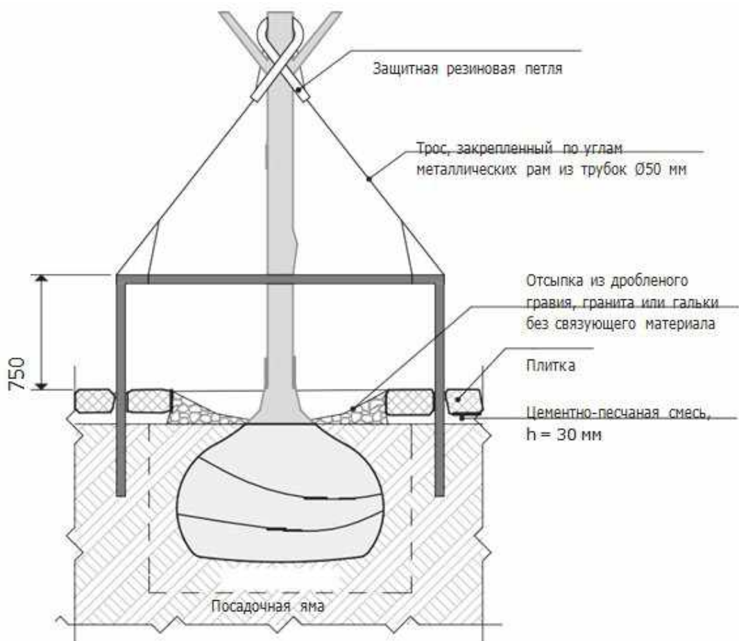
Схема укрепления дерева металлической рамой
