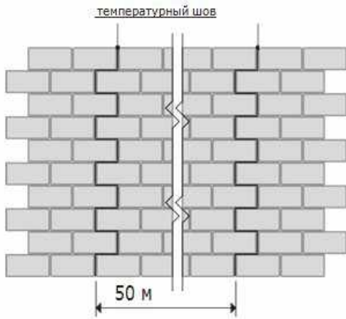
Тип 2. Штабельная перевязка Используемая плитка – прямоугольная
