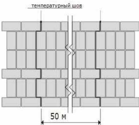
Тип 4. Смешанная ложковая и штабельная перевязка Используемая плитка – прямоугольная
