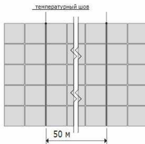
Тип 3. Штабельная перевязка Используемая плитка – квадратная
