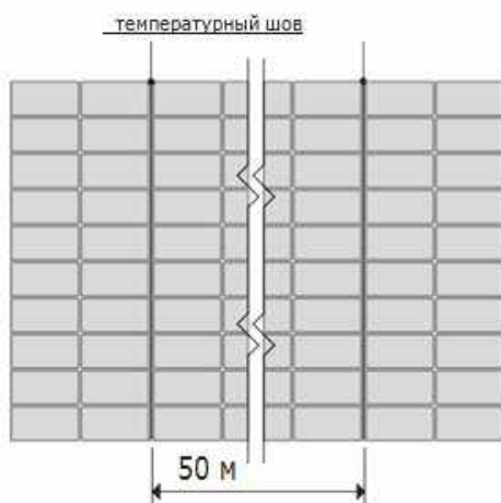
Тип 4. Смешанная ложковая и штабельная перевязка Используемая плитка – прямоугольная
