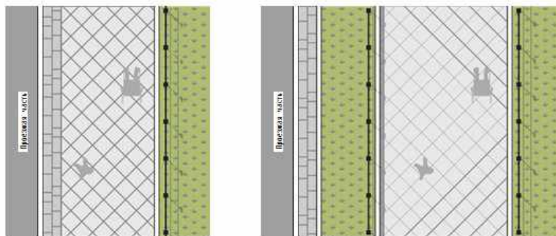
Примеры размещения ограждающих конструкций
