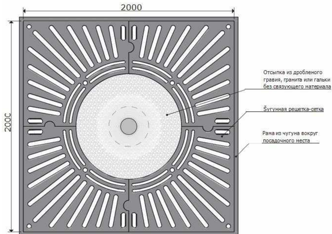
Узел 3.1. Принципиальная схема устройства защиты посадочного места дерева квадратной чугунной решеткой
